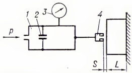
Рис. 2. Пневматический измерительный прибор манометрического типа: 1 — рабочая камера; 2 — входное сопло; 3 — манометр; 4 — измерительное сопло; S — зазор между деталью и измерительным соплом; L — измеряемый размер.
